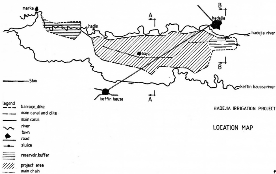
Figuur 3. Schematische weergave van het irrigatie- en drainage systeem in de Hedejia vallei (Brouwer, 1983)
